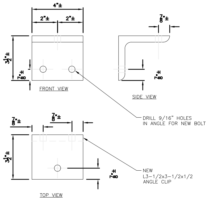
5 ANGLE DETAIL A-7.2 SCALE: NTS
