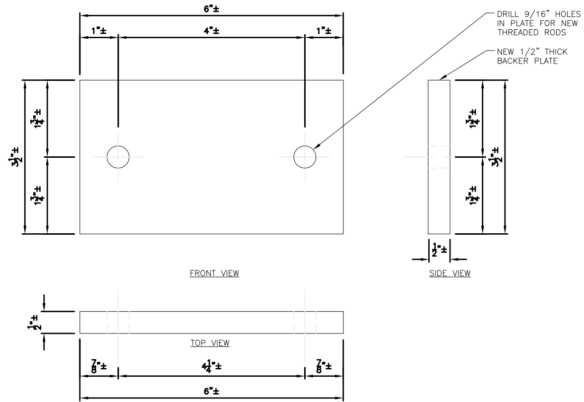
1 STEEL BASE PLATE A-7.2 SCALE: NTS
