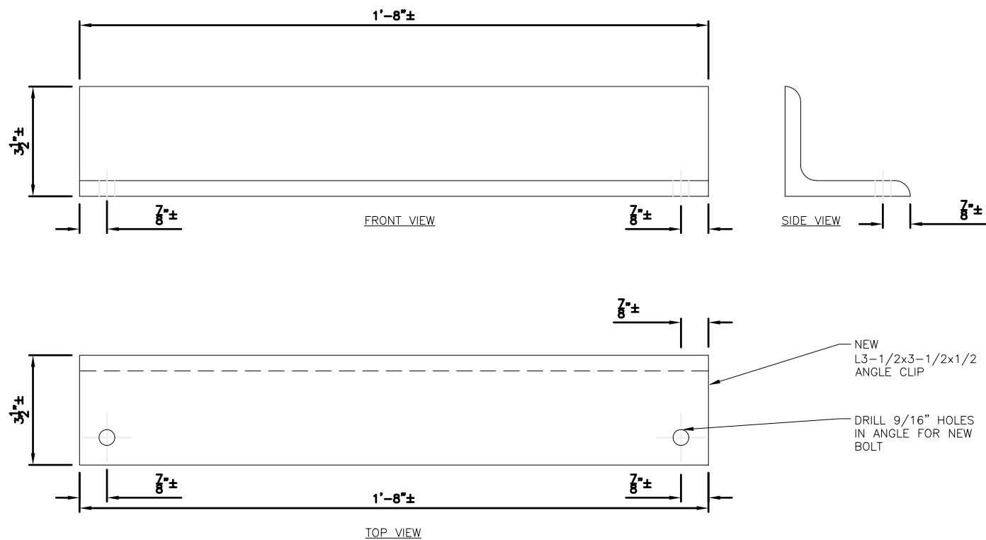
4 ANGLE DETAIL A-7.2 SCALE: NTS
