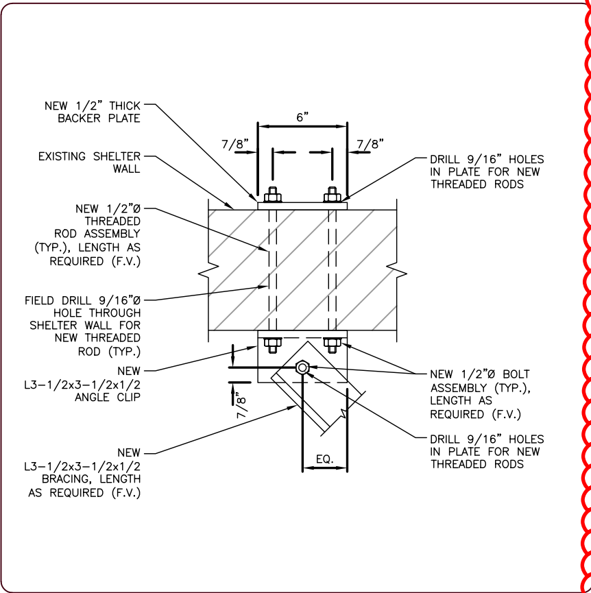
6 SECTION A-7.1 SCALE: NTS
