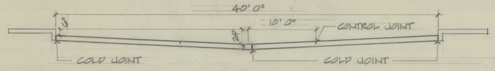
A-A SECTION
