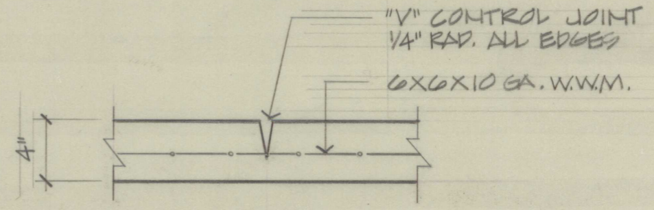
B-B SECTION (TYP.)
