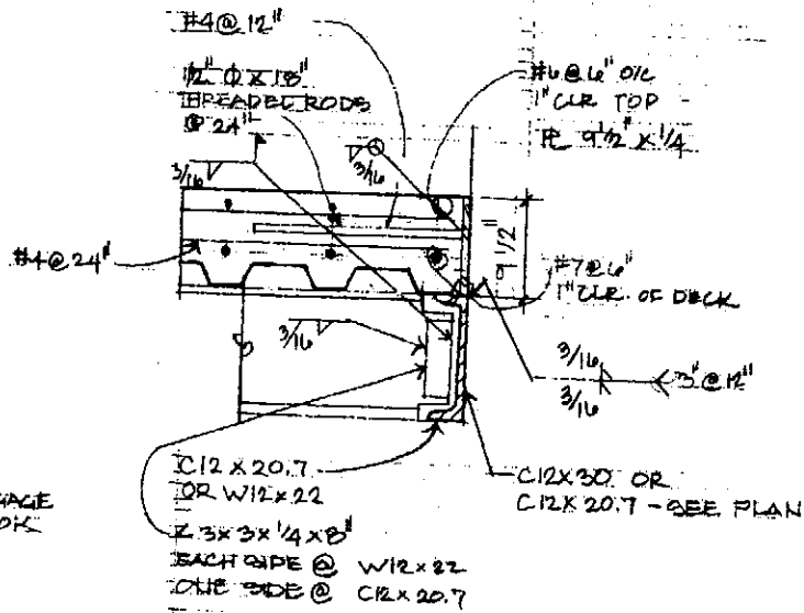
CD2 DETAIL 5/3 SCALE: 1" = 1'-0"
