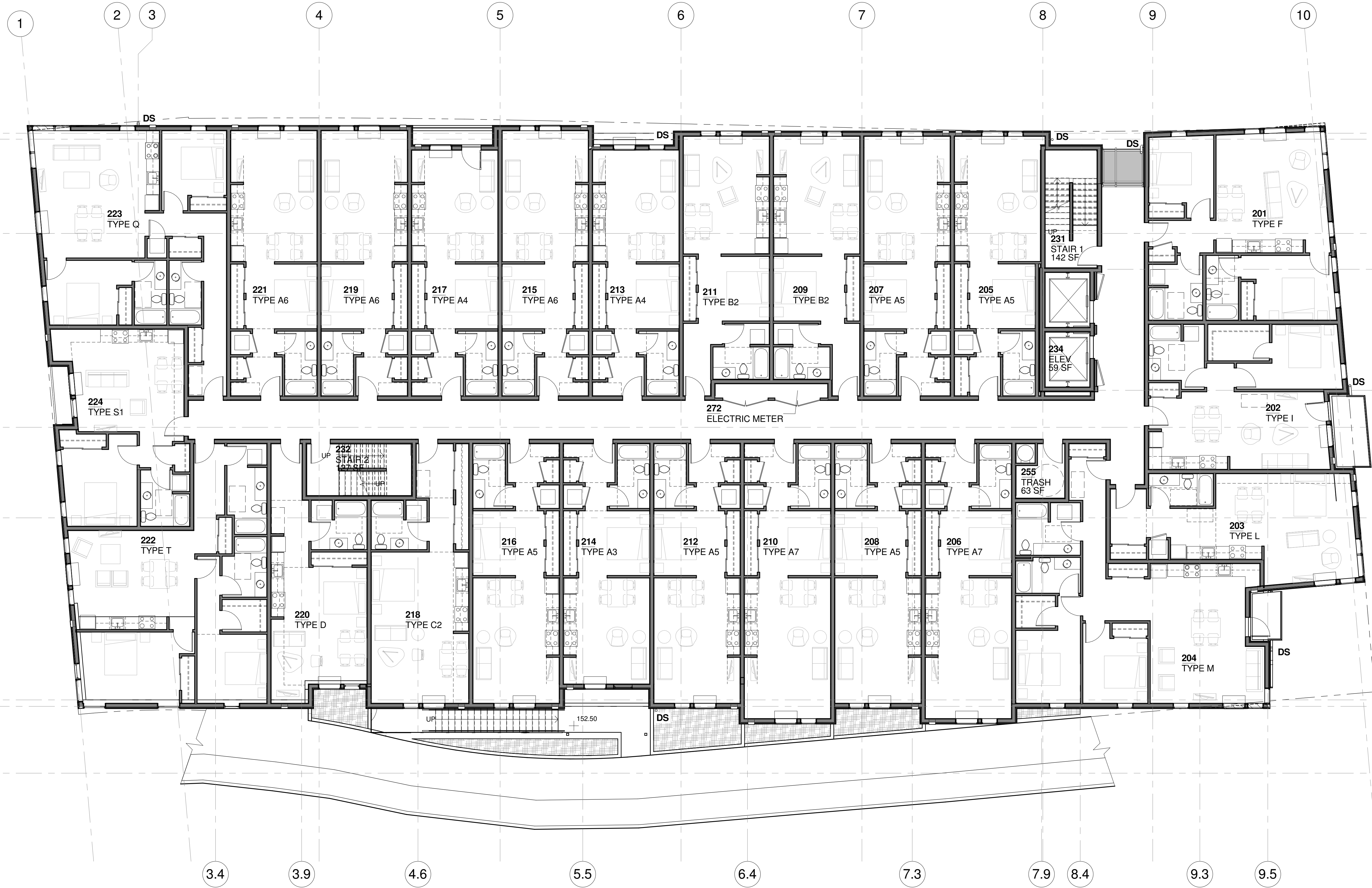
C2.5 | LEVEL 2 1 SCALE: 1/8" = 1'-0"
